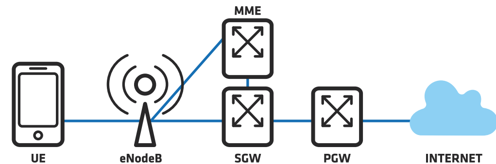
FIGURA 2: ARQUITECTURA SAE BÁSICA
