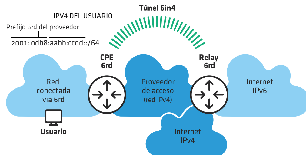
FIGURA 6: TÚNEL AUTOMÁTICO 6RD
