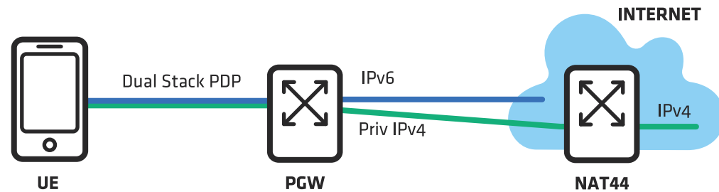
FIGURA 5: IMPLEMENTACIÓN DE DUAL STACK
