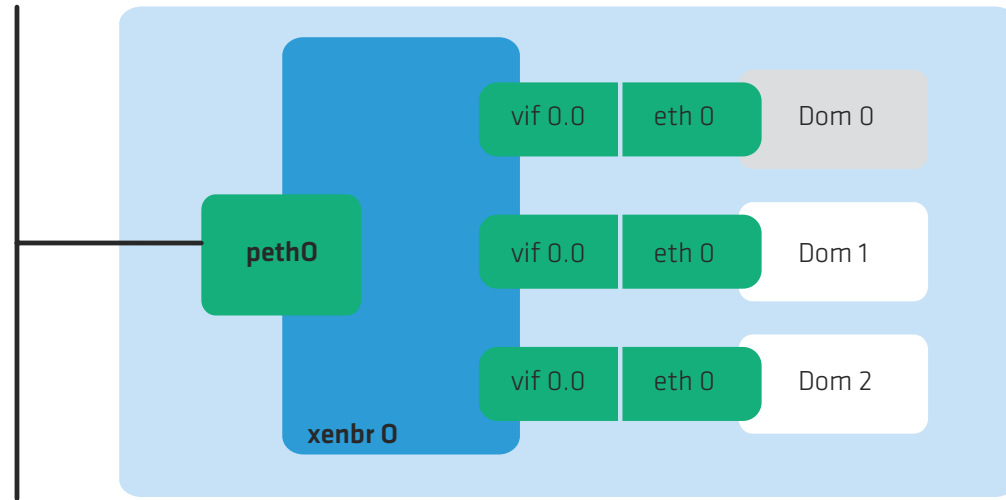
FIGURA 8: XEN EN MODO BRIDGE
