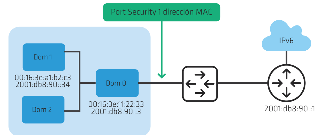
FIGURA 7: ESCENARIO PROXY NDP
